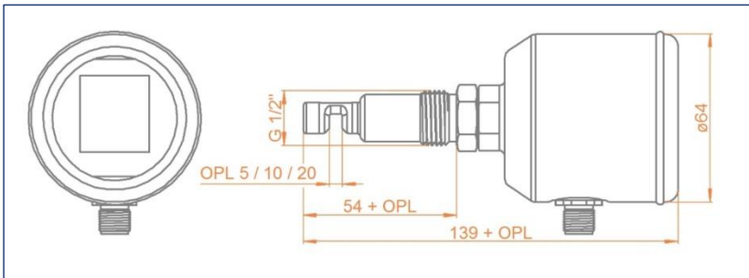
Abb. 1: Abmessung Sensor
