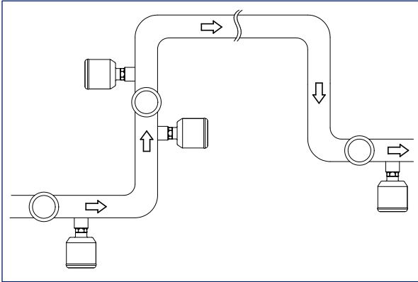
Abb. 6: Einbaulagen
