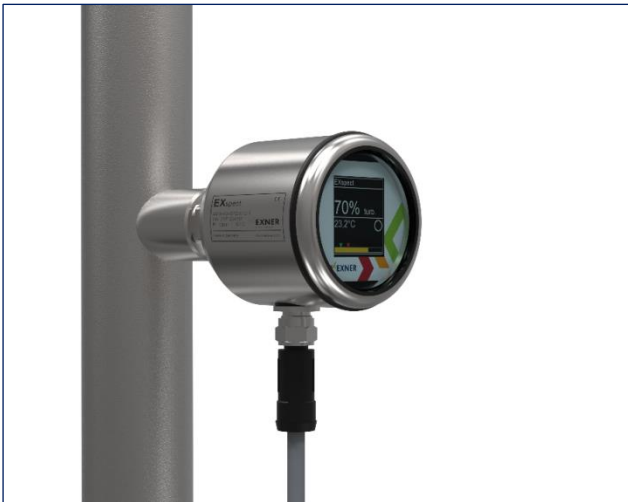
Abb. 5: Prozessintegration
