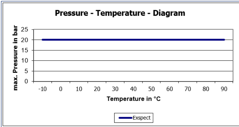
Abb. 2: Druck-Temperatur-Diagramm EXspect 271
